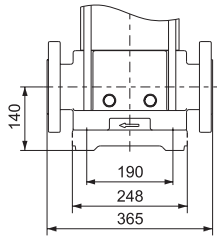
DIN FLANGE(LVR)/F
