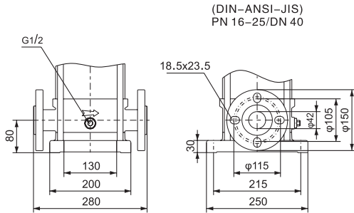
DIN FLANGE(LVS)/F
