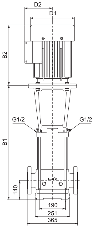
DIN FLANGE(LVS)/F
