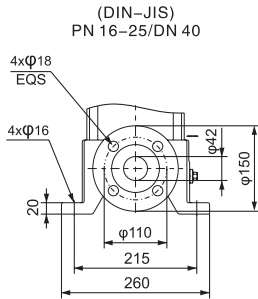
DIN FLANGE(LVR)/F
