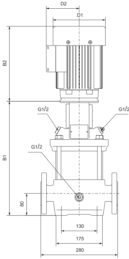
DIN FLANGE(LVR)/F
